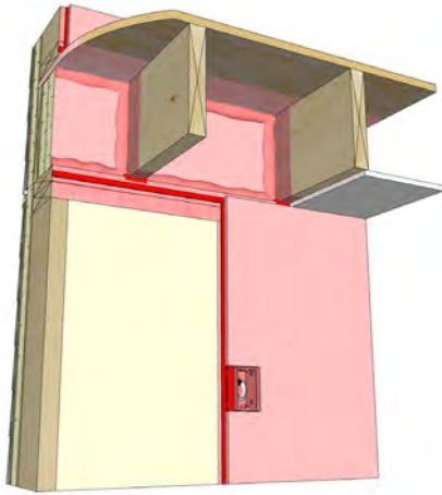
Airtight Drywall
